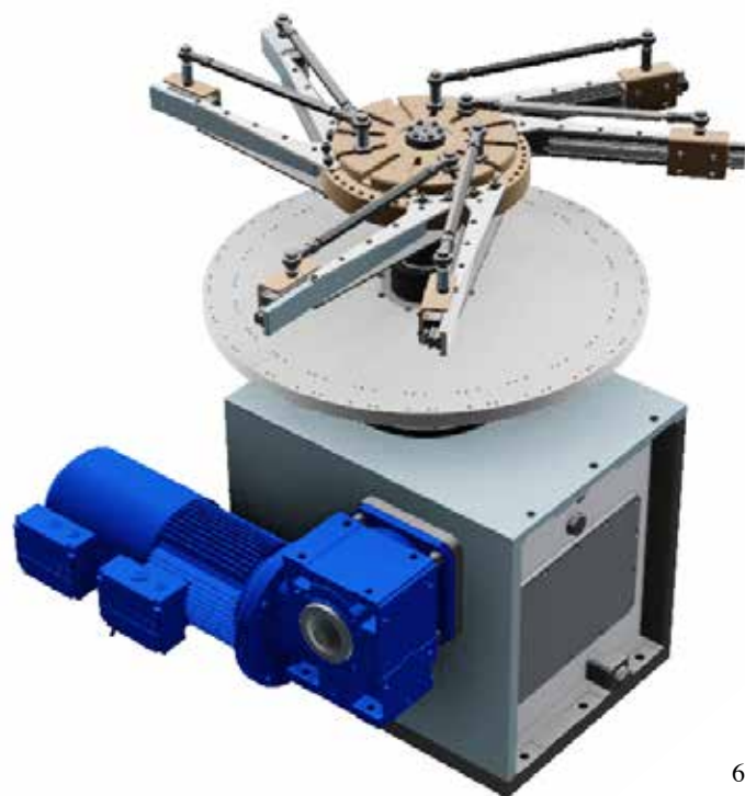
Dispositivo a camme per pick & place.
